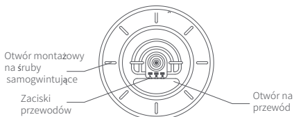
Płyta podstawy
