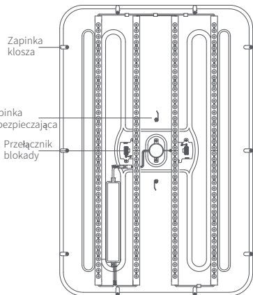
Płyta podstawy
